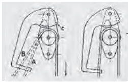
Seilblockierungssystem
